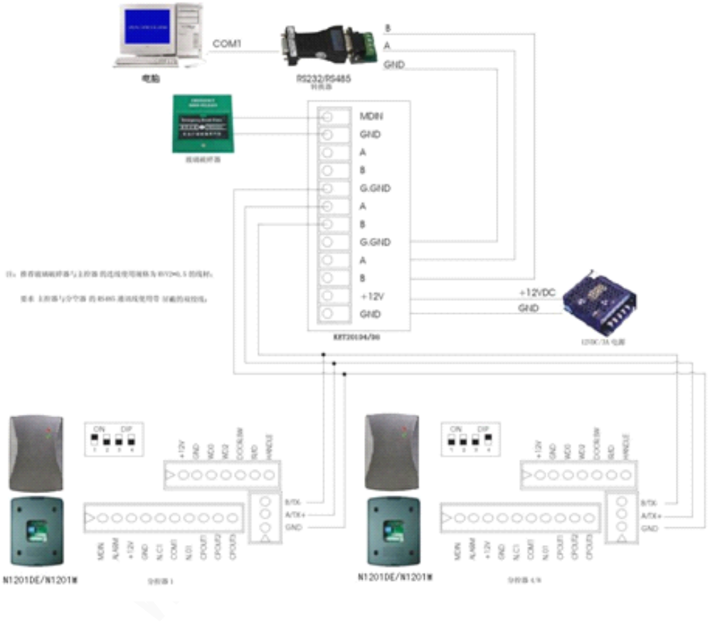
N1201D4/N1201D8接线图
